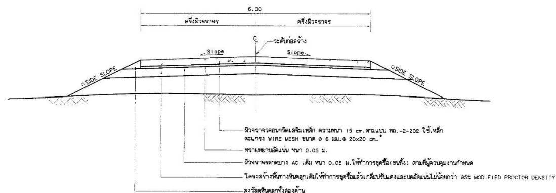
แบบรูปตัดโครงสร้างทาง
