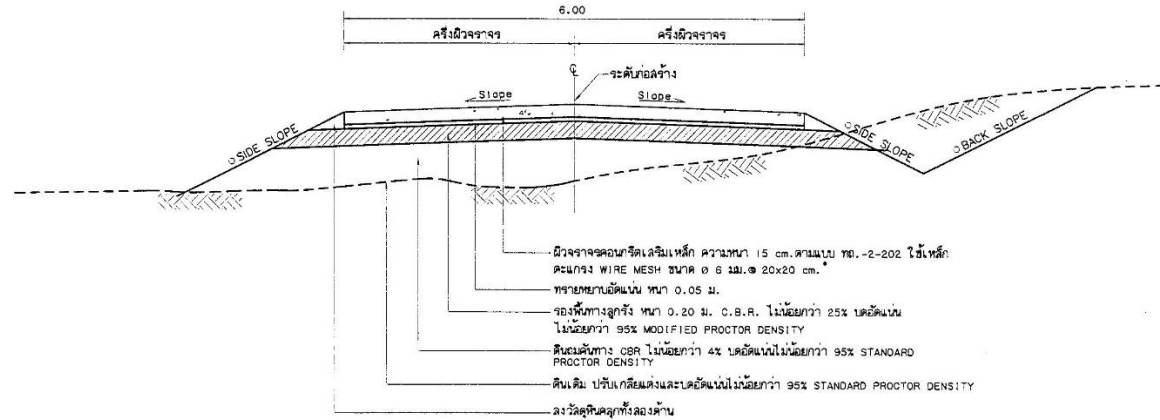
แบบรูปตัดโค้งสร้างทาง
